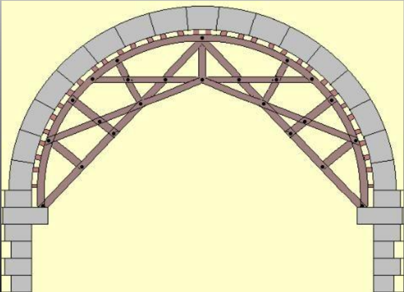
CIMBRA EN ARCOS
